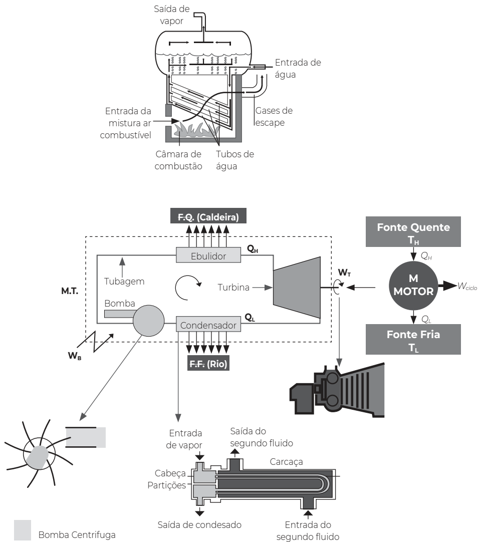
FIG. 6.5. Central térmica. Adaptado de [8].
