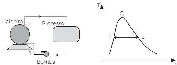
FIG. 11.2. Produção de calor para um processo.
