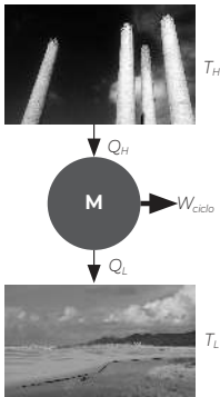
FIG. 10.1. Máquina Térmica Motora.
