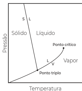
FIG. 4.7. Superfície p - T da água. Adaptado de [4].
